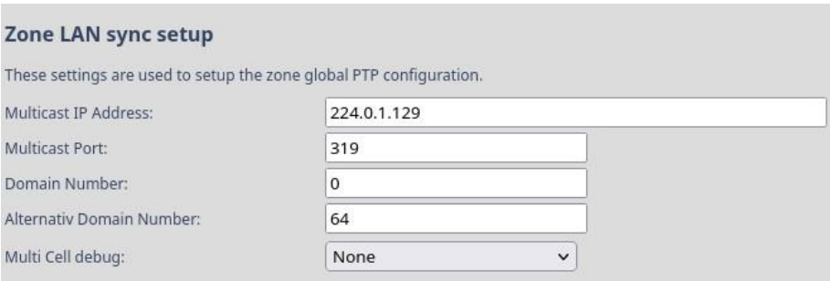
Figure 4: LAN sync setup
